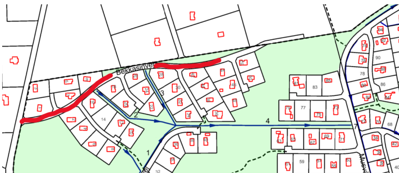
Figur 1 Stamvej markeret med rødbrun streg. Grøfter markeret med blå streg.
